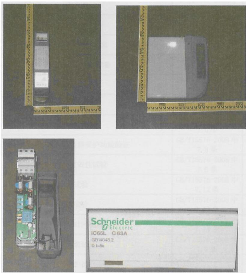
铭牌
